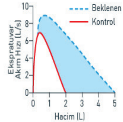
FEV 1 /FVC (%)
